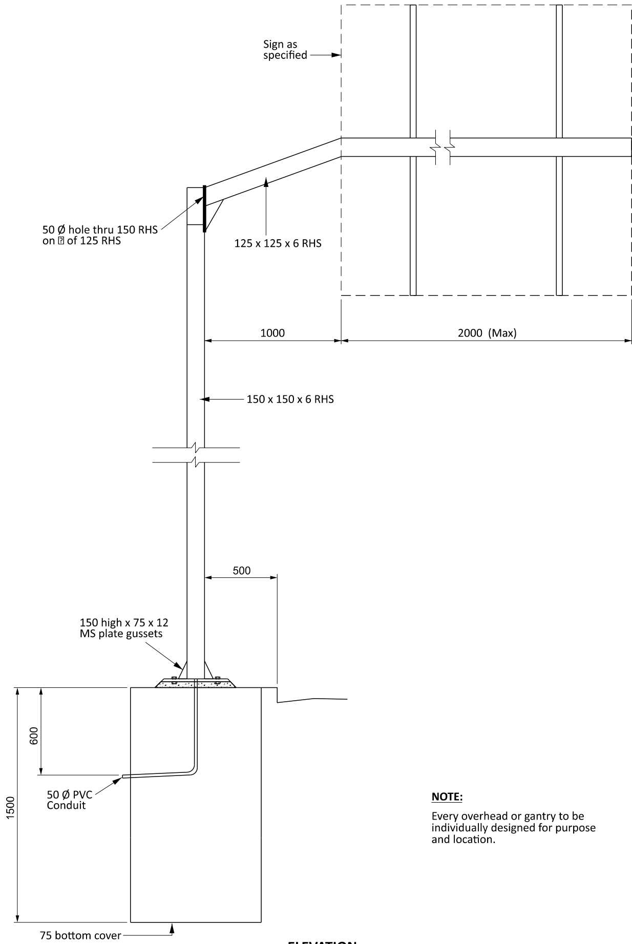
ELEVATION
