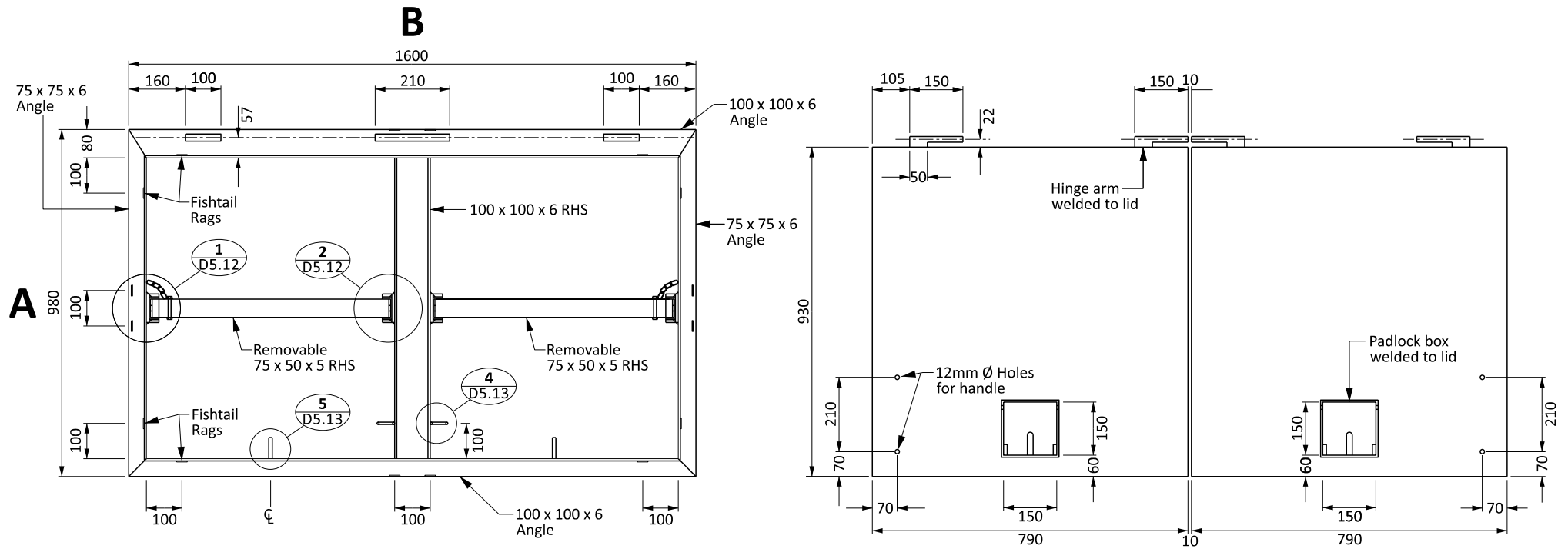
FRAME FOR DOUBLE LID (Flygt 3127 & 3153 Pumps)
